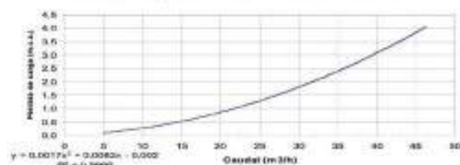
Pérdida de carga filtro de anillo de 140 Mesh de 3". Ref: 2160
