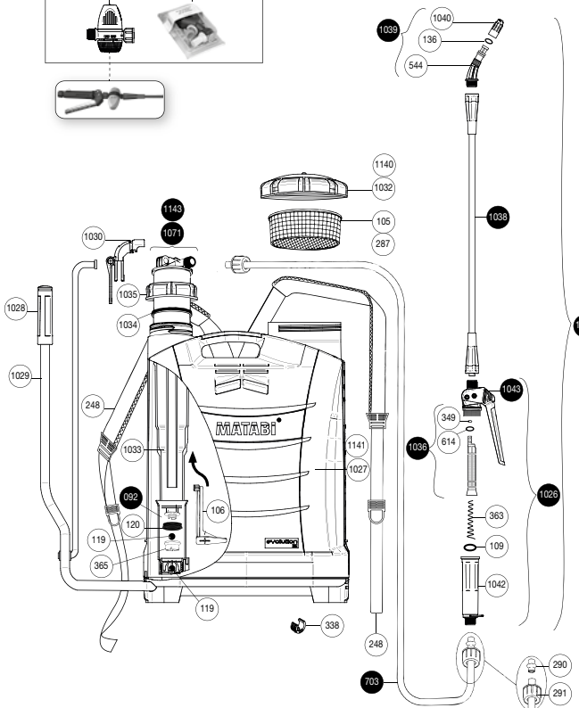
TUBO DE LANZA DE 1M ALUMINIO CON CODILLO COMPLETO cod. 8.34.60.871 TUBO DE LANZA DE 1,5 M ALUMINIO CON CODILLO COMPLETO cod. 8.34.60.872
