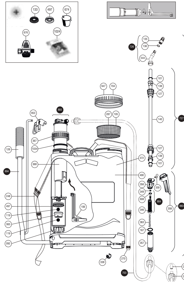
TUBO DE LANZA DE 1M ALUMINIO CON CODILLO COMPLETO cod. 8.34.60.871 TUBO DE LANZA DE 1,5 M ALUMINIO CON CODILLO COMPLETO cod. 8.34.60.872
